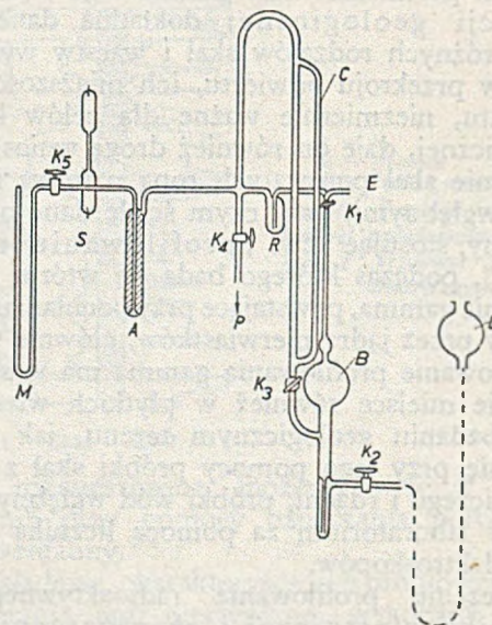
A — adsorber z węglem aktywnym, B — miernica manometru, C — kapilara miernicza, E — wlot gazu badanego, K 1 — kurek trójdrożny, K 2 , K 3 , K 4 , K 5 — kurki normalne przelotowe, R — łapacz rurek do kontroli widma gazu.
