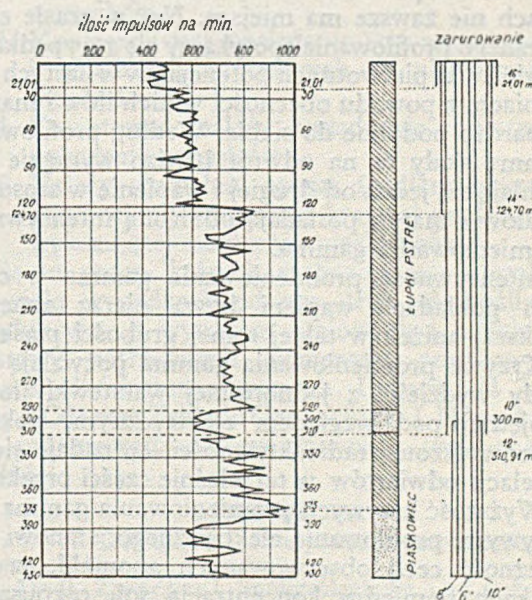
Rys. 4. Wynik pomiaru promieniotwórczości skał w odwiercie naftowym
