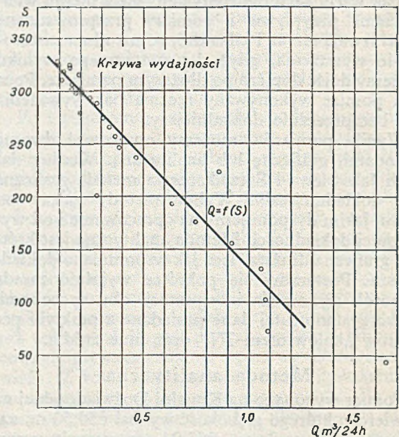
Rys. 2. Krzywa wydajności obliczona analitycznie
