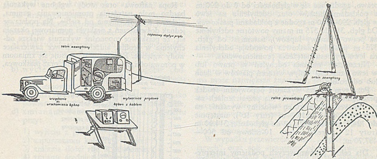
Rys.3. Rozstaw urządzeń do badania promieniotwórczości w odwiercie
