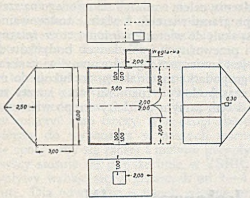
Rys. 5. Kuznia kopalniarna mniejsza
