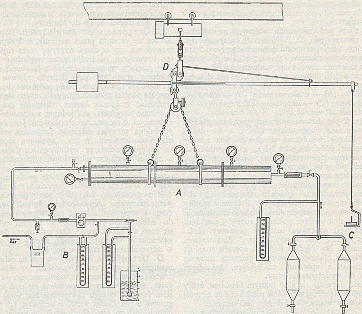
A—złożo właściwe, B—aparatus do napełniania, C—urządzenia odbiorcze, D—urządzenie dźwigowe Rys. 1. Schemat aparatury „sztuczne złożo”
