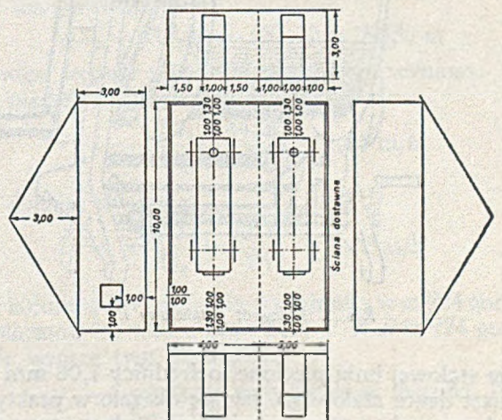
Rys. 6. Kotłownia wielokotłowa
