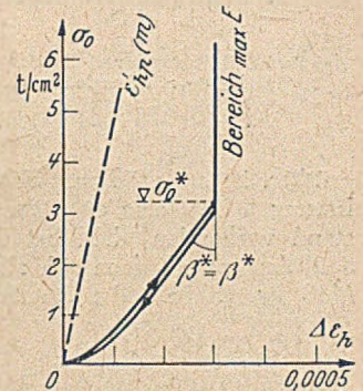
Abb. 13. Schematische Darstellung der Dehnungsunterschiede.
