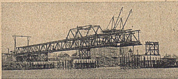
Abb. 12. Die Montagespitze kurz vor Erreichen eines Pfeilers.
