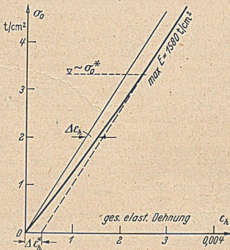
Abb. 12. Die elast. Längsdehnung \varepsilon_h und die Hooke'sche Gerade für den „Bereich der Verkehrslasten“. (schematisch für s = 10,25 .)
