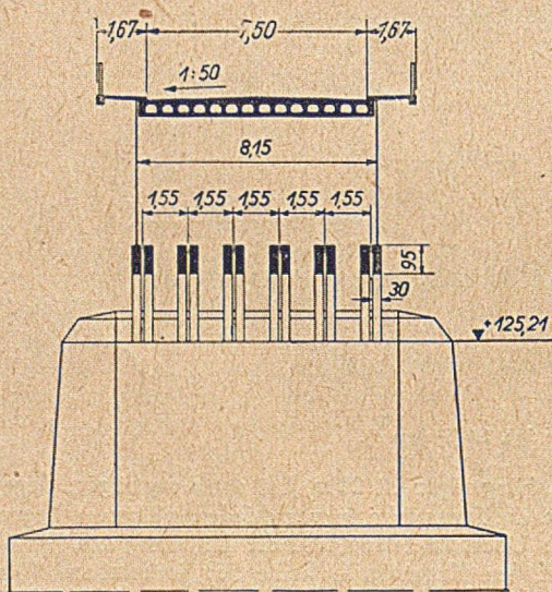
Abb. 2. Längs- und Querschnitt durch die Brücke.
