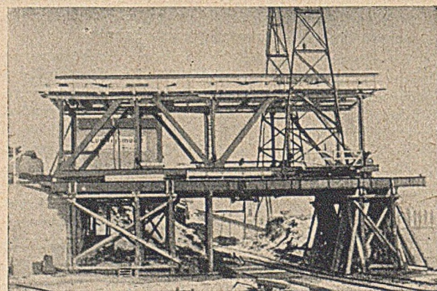
Abb. 3. Montage der landseitigen Hälfte des 48-m-Überbaus auf festem Gerüst.
