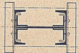
Abb. 4. Behelfsmäßige Aussteifung der Pfosten 2, 4, 4', und 2'.
