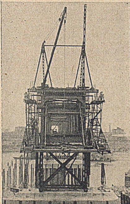
Abb. 6. Der Freivorbauerrück mit Montageschutzpodium beim Überschreiten eines Pfeilers.
