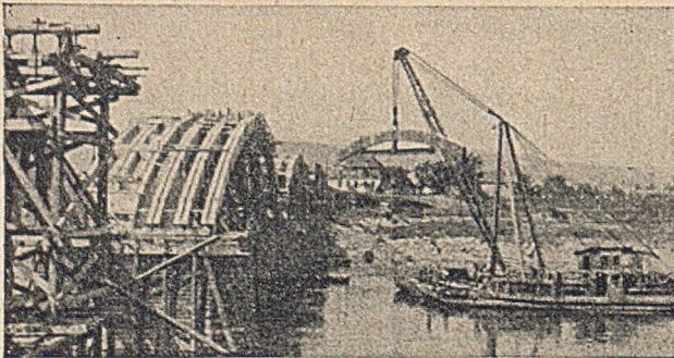
Abb. 13. Versetzen eines Werkstückes durch den Schwimmkran.
