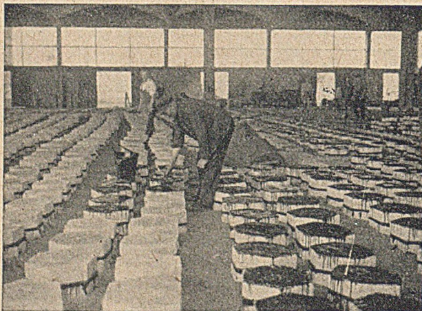
Abb. 2. Sechseckplatten. Aufbringen des Kaltasphaltanstriches.
