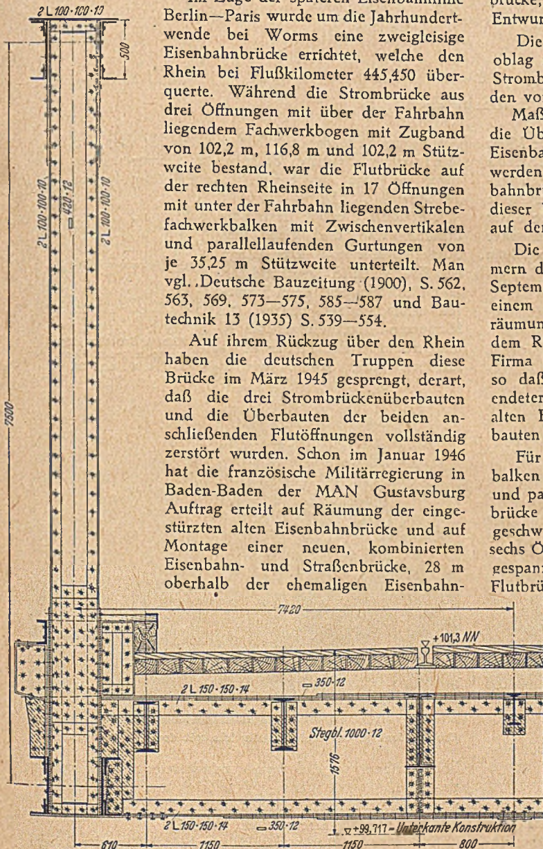
Abb. 2. Normaler Brückenquerschnitt.
