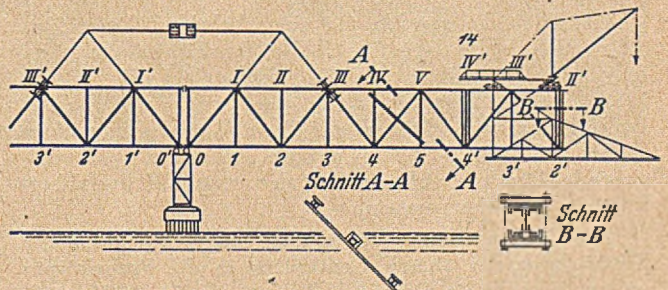
Abb. 14. Unterteilung der Knicklänge der Diagonale 4-V und Aussteifung der Pfosten 4' und 2'.
