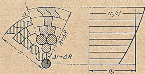
Abb. 15. Links: Querverföderung. Rechts: Spannungsumlagerung für \sigma_0 < \sigma_0^* .
