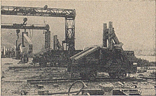
Abb. 11. Verladen der Werkstücke auf die Hunde der Ablaufbahn.
