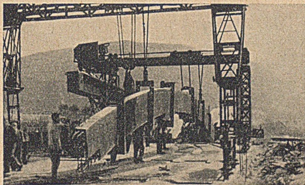
Abb. 8 bis 10. Drehung der Fertigstücke.
