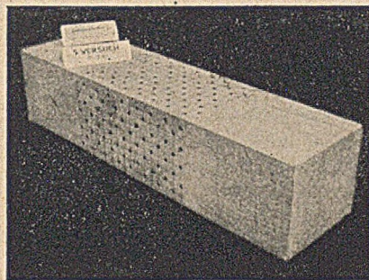
Abb. 3: Versuch 5: Beide Druckflächen und beide Seitenflächen genagelt.
