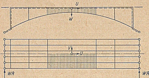
Abb. 4. Ableitung der Windkräfte aus der Fahrbahn in die Pfeiler.
