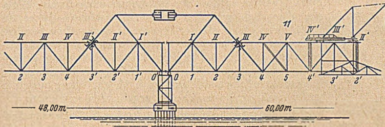
Abb. 11. Schematische Darstellung des Abspanngerätes.
