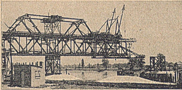
Abb. 10. Das Abspanngerät in Tätigkeit.
