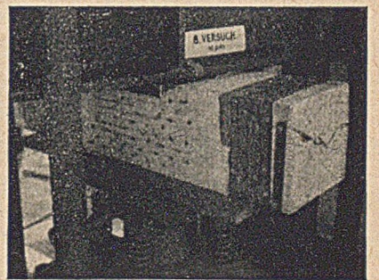
Abb. 6: Versuch 8 bei 30 mm Eindrückung.
