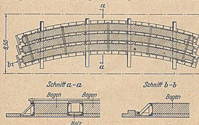
Abb. 6. Die Schalungsform für die Bogenstücke.
