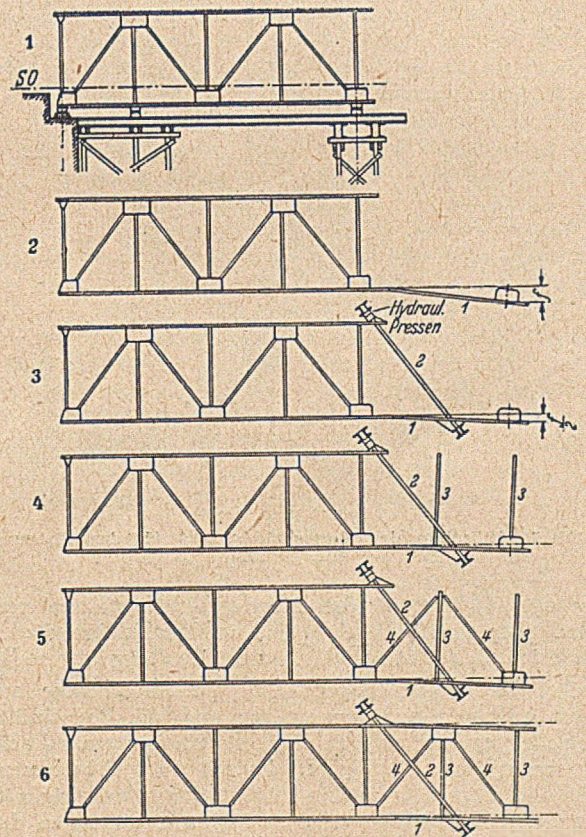
Abb. 8. Schematische Darstellung der Montagefolge eines doppelten Brückenfeldes.
