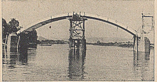
Abb. 14. Montagegerüst.
