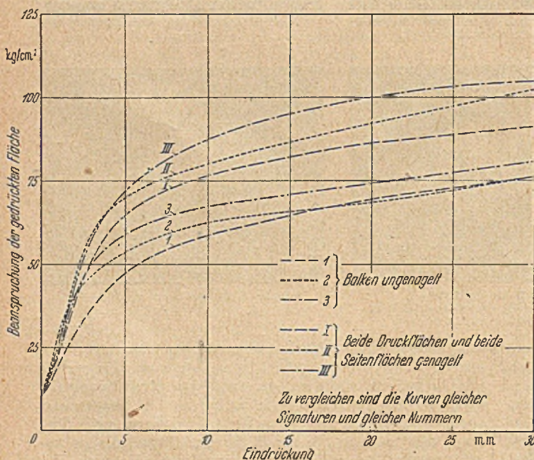
Abb. 8: Spannungs-Eindrückungs-Diagramme von vergleichsfähigen ungenagelten und allseitig genagelten Probekörpern.
