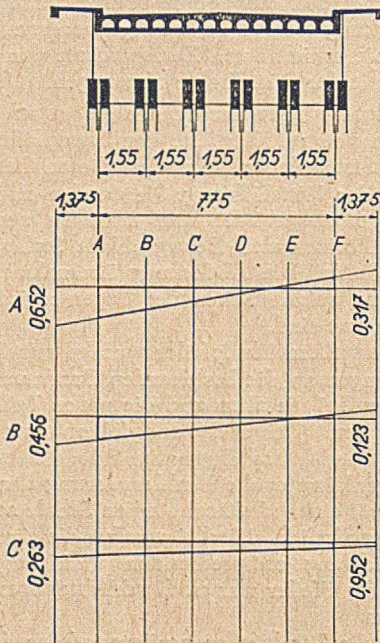
Abb. 3. Einflußlinien für die querverteilende Wirkung der Fahrbahnunterstützung.
