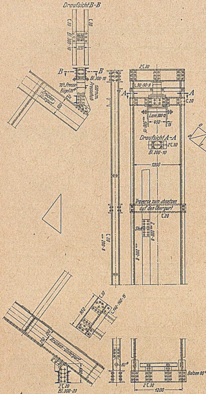
Abb. 7. Hilfsdiagonale (Montagerückhaltung) für den Einbau der Untergurtstäbe.
