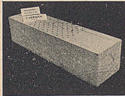
Abb. 1: Probekörper zu Versuch 2: Obere Druckfläche genagelt.
