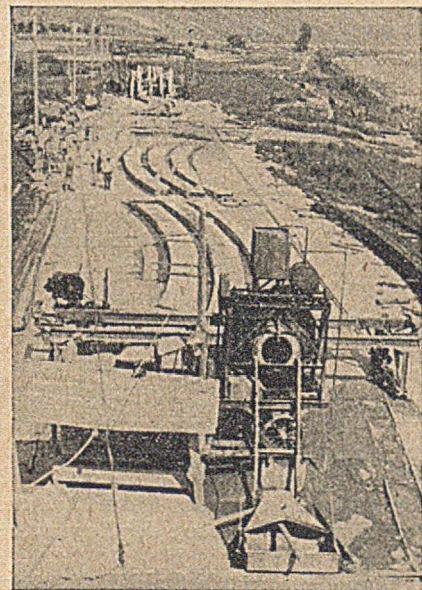
Abb. 5. Einrichtung des Werkplatzes zur Herstellung der Fertigbetonteile.
