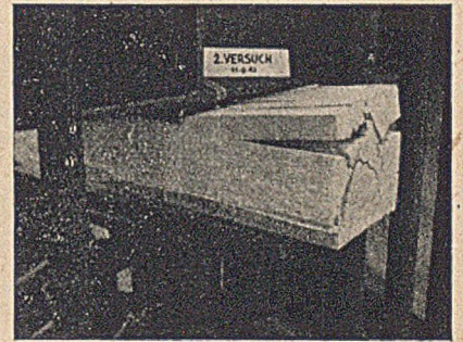
Abb. 2: Versuch 2 bei 30 mm Eindrückung.
