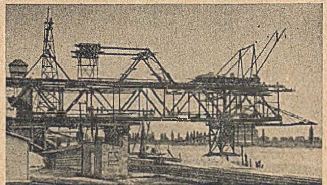
Abb. 9. Montage der beiden ersten Felder des ersten 60-m-Überbaues und Montage des Abspanngerätes über dem 48-m-Überbau.
