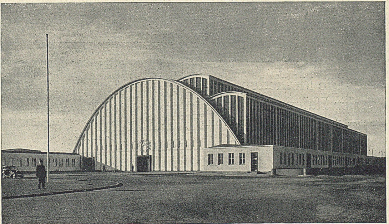
GROSSMARKTHALLE KÖLN SCHALENBÄUWEISE SYSTEM ZEISS-DYWIDAG
