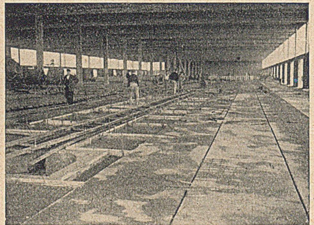
Abb. 4. Fußbodenplatten 1,50 \times 2,00 m.
