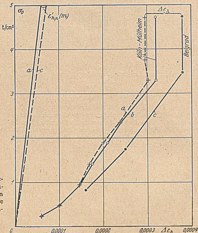
Abb. 16. Abschätzung der Querverföderung.
