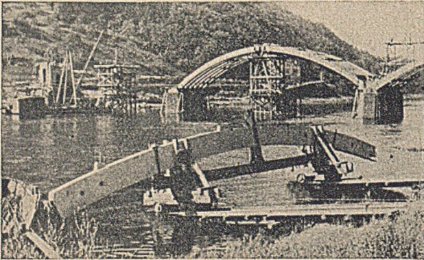
Abb. 12. Das Werkstück ist am Wasser angekommen.
