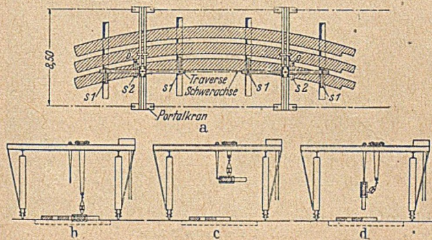
Abb. 7. Vorrichtung zum Aufheben und Drehen der Fertigbetonstücke.
