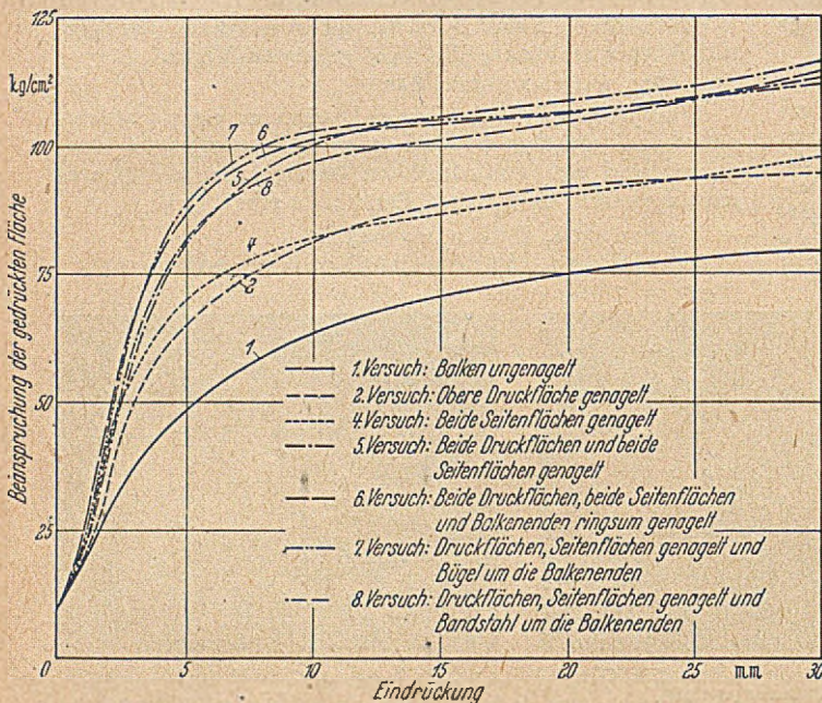
Abb. 7: Spannungs-Eindrückungs-Diagramme einer Versuchsreihe (8 Versuche mit verschiedenen Anordnungen).
