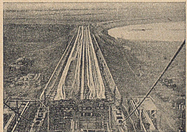
Abb. 18b. Seilreckbahn Savebrücke Belgrad. (Nach Roß [12] Abb. 145.)
