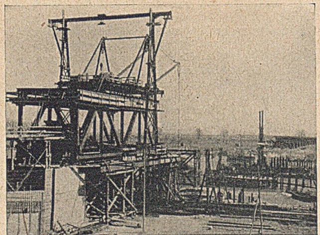
Abb. 5. Montage des Freivorbauerricks mit dem Montageportalkran.
