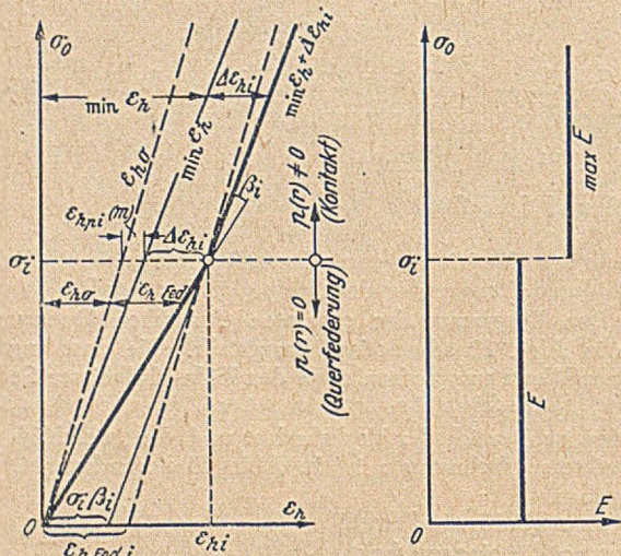
Abb. 14. Dehnungen und Elastizitätsmodul für eine einzelne Drahtlage - mit Querverföderung. Gesamte Längsföderung
