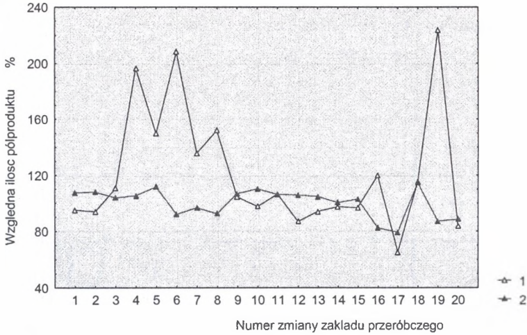
Rys. 5. Względne ilości półproduktu (odniesione do ilości półproduktu przy stałej charakterystyce nadawy i zadanych gęstościach cieczy ciężkich): 1 – przy zmierzonych gęstościach cieczy ciężkich, 2 – przy średnich gęst. cieczy ciężkich
