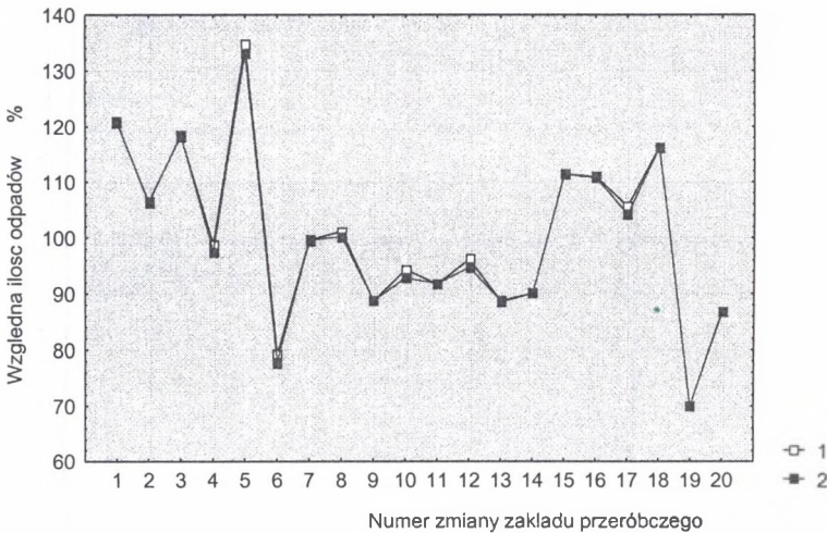
Rys. 6. Względne ilości odpadów (odniesione do ilości odpadów przy stałej charakterystyce nadawy i zadanej gęstości cieczy ciężkiej 1,78 g/cm 3 ): 1 – przy zmierzonych gęst. cieczy ciężkich, 2 – przy średnich gęst. cieczy ciężkich
