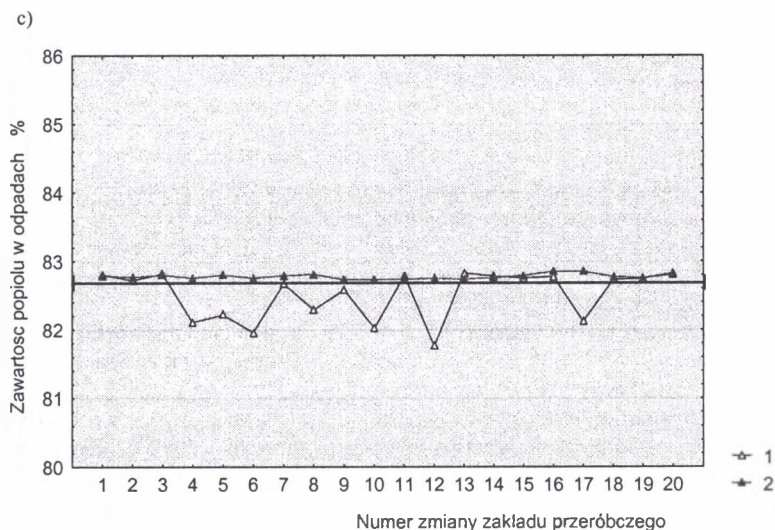
Rys. 7. Średnie zawartości popiołu w poszczególnych zmianach roboczych zakładu przerobczego: a) w koncentracji, b) w półprodukcie, c) w odpadach; 1 – przy zmierzonych gęst. cieczy ciężkich, 2 – przy średnich gęst. cieczy ciężkich
