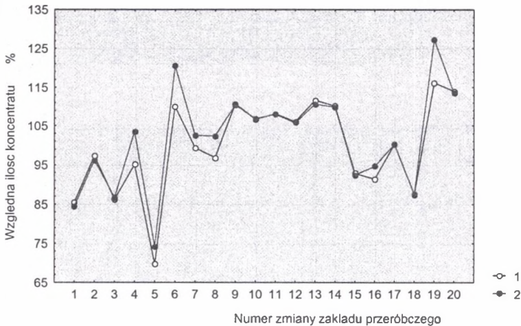
Rys. 4. Względne ilości koncentratu (odniesione do ilości koncentratu przy stałej charakterystyce nadawy i zadanej gęstości cieczy ciężkiej 1,48 \text{ g/cm}^3 ): 1 – przy zmierzonych gęstościach cieczy ciężkiej, 2 – przy średnich gęst. cieczy ciężkiej
