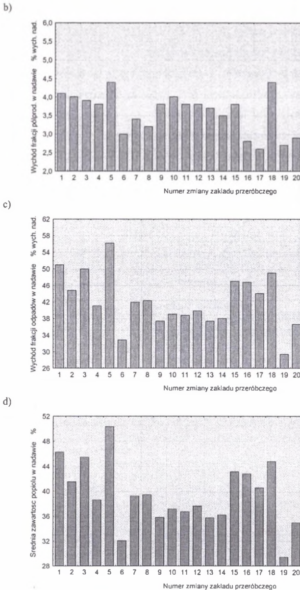
Rys. 2. Wychody frakcji koncentratu (a), półproduktu (b), odpadów (c) oraz średnia zawartość popiołu w nadawie (d) w poszczególnych zmianach roboczych zakładu przerobczego
