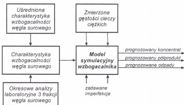
Rys. 1. Idea metody prognozowania efektów wzbogacania wzbogacalnika zawieszinowego, wykorzystująca pomiary gęstości cieczy ciężkich
