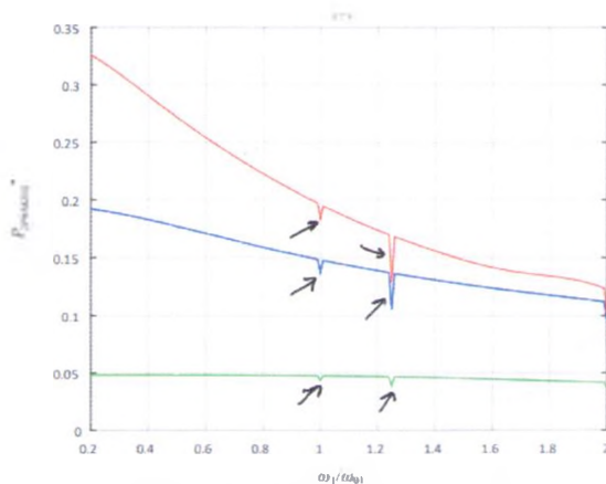
Rys. 4.16. Charakterystyki sterowania mocy składowej HF w funkcji pulsacji sygnału modulującego dla trzech wartości dobroci Q_2 obwodu 2F [k_n = 0.1, k_i = k_c = 10, M = 0.9, \omega_1/\omega_0 = \text{const} = 5, P_{\text{PWM}} = f(\omega_1)] , wyznaczone z wykorzystaniem względnych impedancji odniesionych do: (a) rezystancji R_2 ; (b) impedancji charakterystycznej Z_0 .
