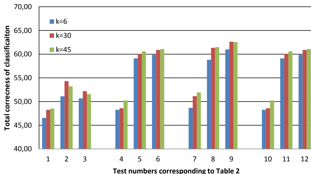
Fig. 1. Results of different normalization methods for the the three best k values Rys. 1. Wyniki dla różnych metod normalizacji dla trzech najlepszych wartości k
