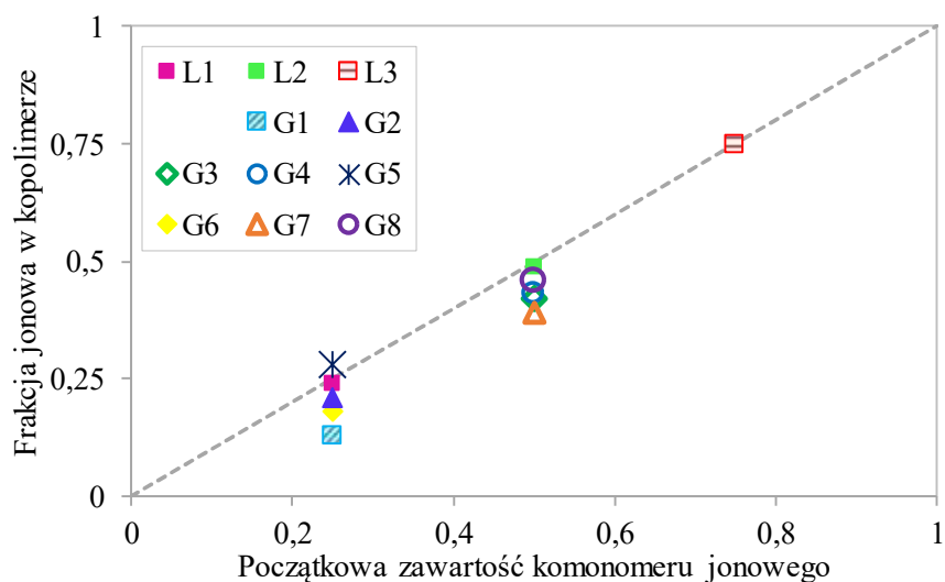
Rysunek 4. Zależność składu kopolimeru od składu początkowego mieszaniny komonomerów.
