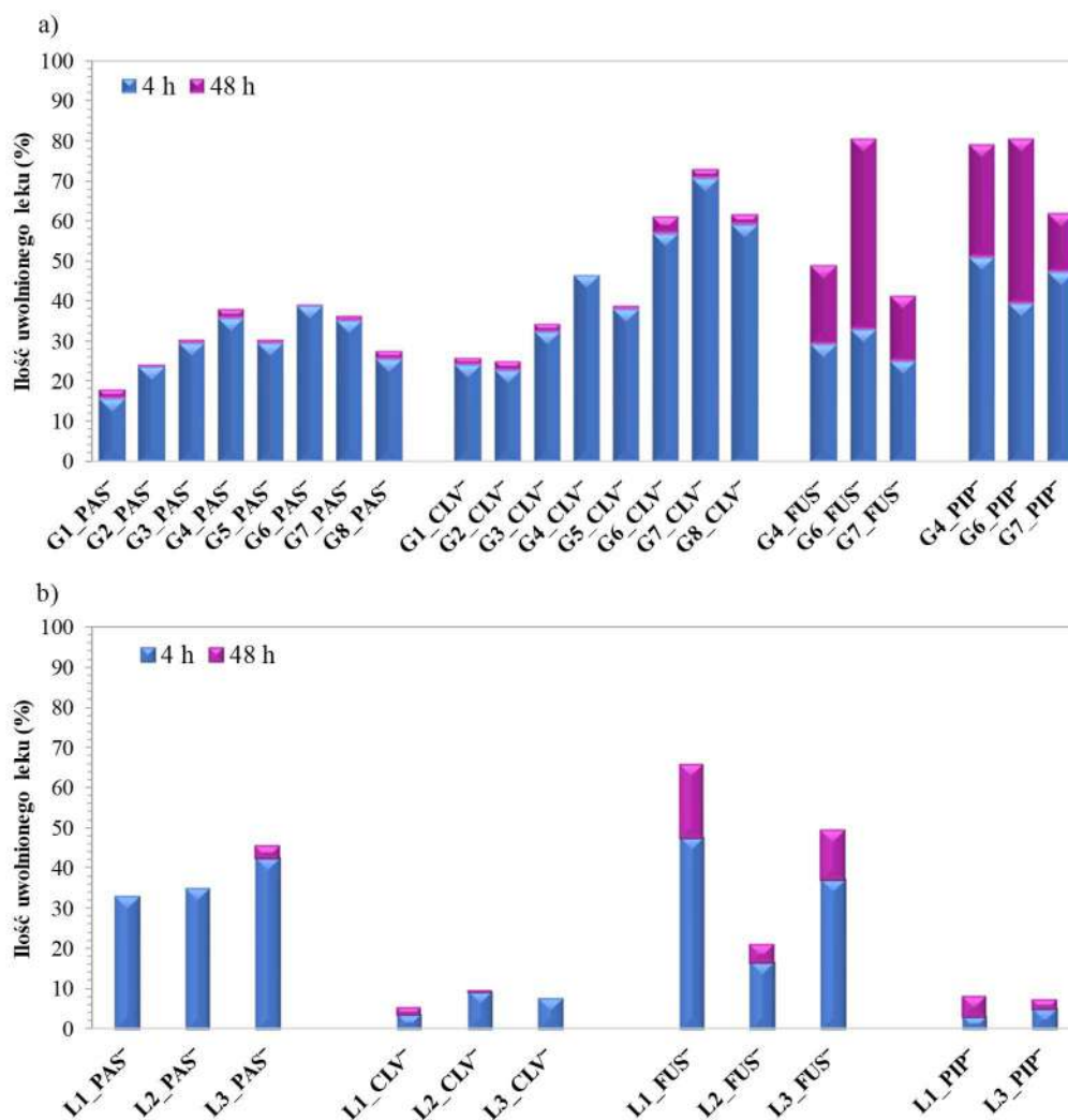
Rysunek 10. Isici uwolnionych leków jonowych dla ukadów a) szczepionych b) liniowych.
