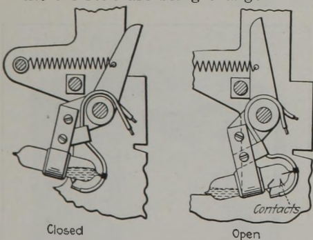
Fig. 3—Mercury Contact Switch
