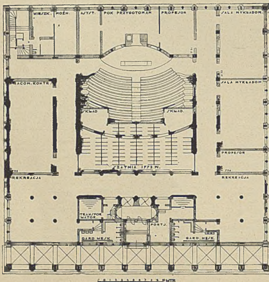
ARCH. JAN WITKIEWICZ. PAWILON ZAKŁADÓW DOŚWIADCZALNYCH W.S.H.
