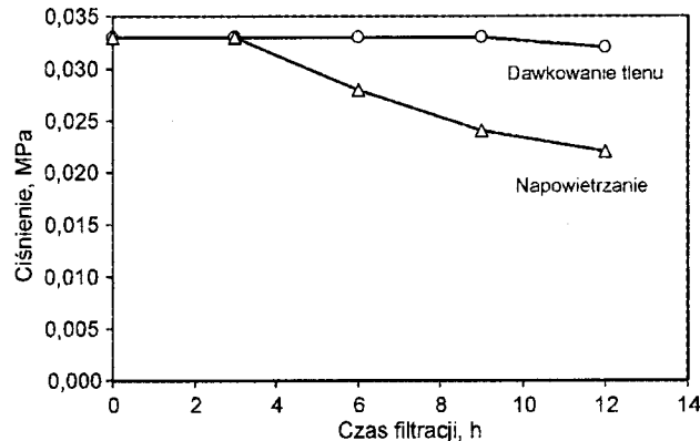
Rys. 3. Zmiany oporów filtracji wody podziemnej
