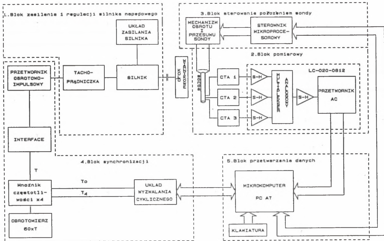
Rys. 8.2. Schemat pomiarowy
