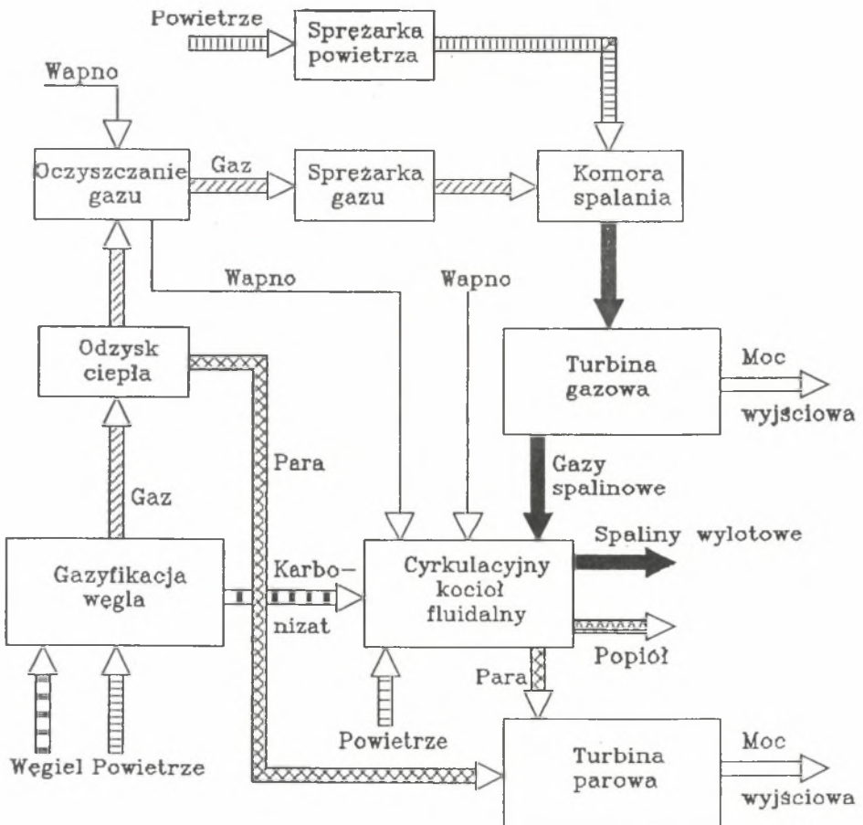
Rys. 7. Układ parowo-gazowy zintegrowany z instalacją pirolizy węgla (technologia IChW). Schemat blokowy
