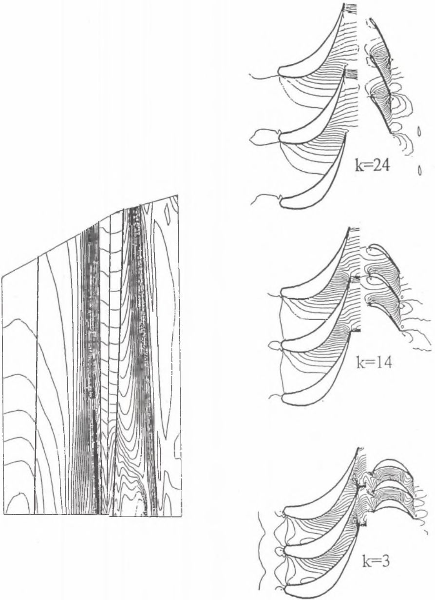
Rys. 3. Rozkład ciśnienia statycznego w stopniu turbiny parowej [10, 11]
