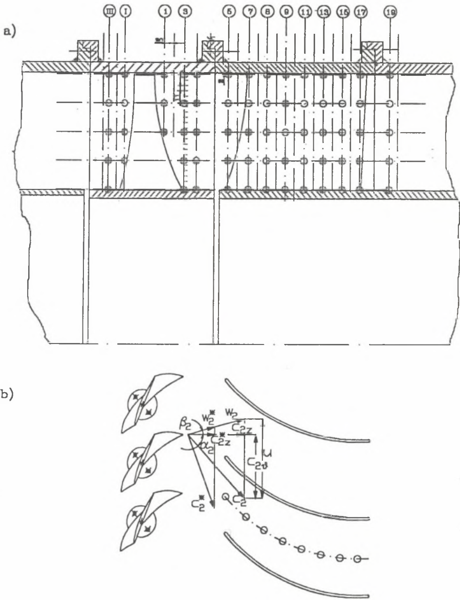
Rys. 8.3. Lokalizacja punktów pomiarowych
