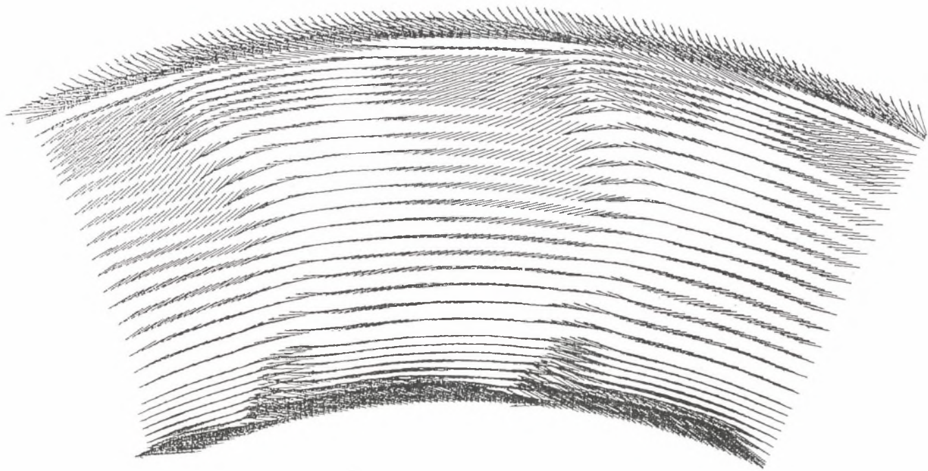
Rys. 8.5. Pomiar przepływów wtórnych
