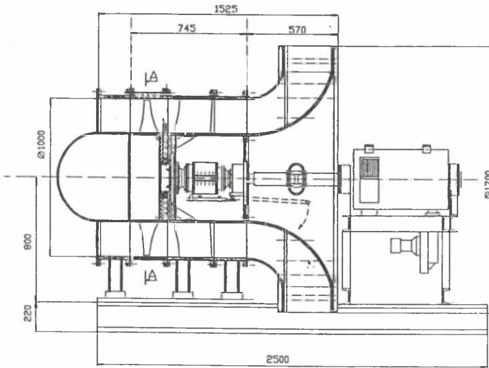
Rys. 8.1. Ogólny schemat wentylatora badawczego
