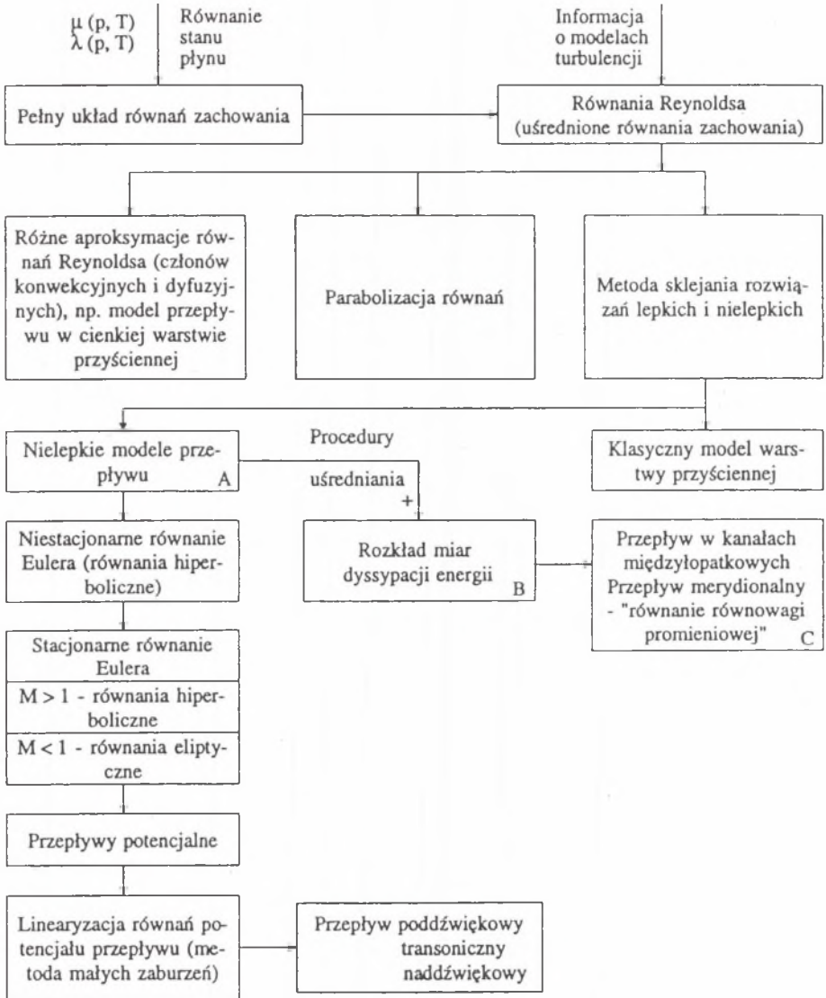
Rys. 1. Modelowanie przepływów w maszynach wirnikowych
