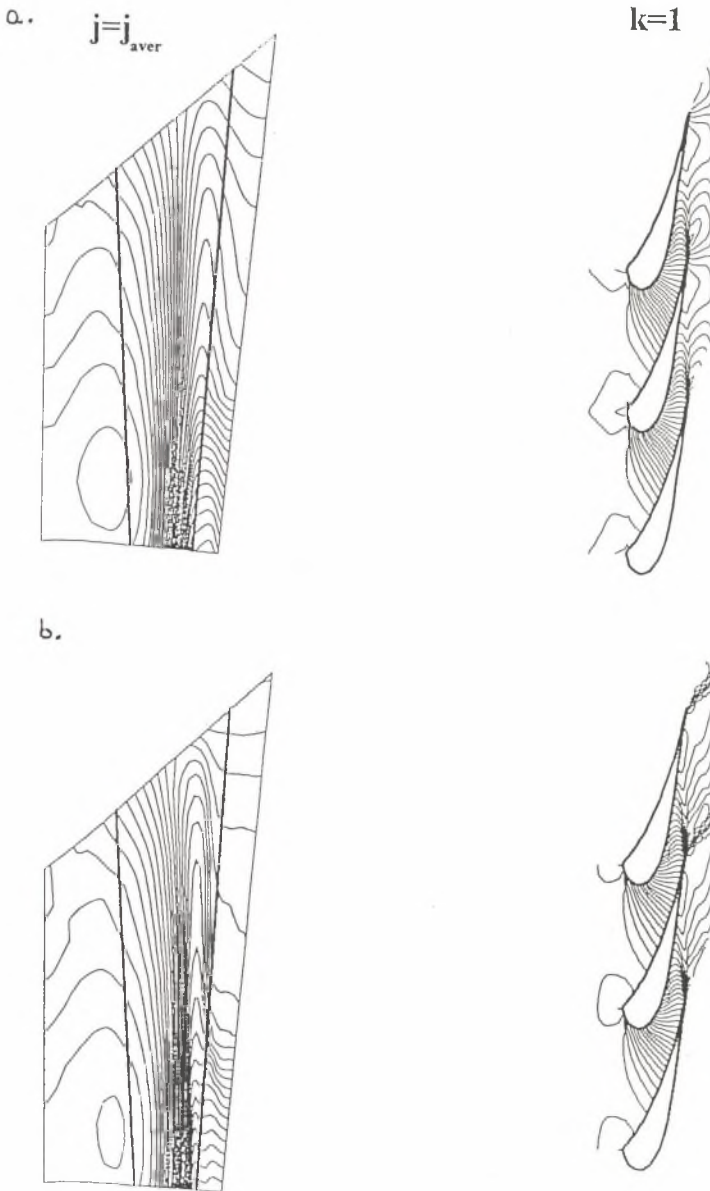
Rys. 2. Rozkład izobar dla kierownicy [10, 11]: a. Schemat pierwszego rzędu dokładności, b. Schemat trzeciego rzędu dokładności
