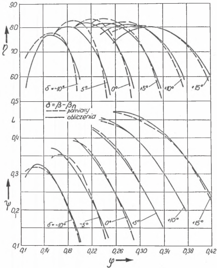
Rys. 6. Porównanie charakterystyk obliczeniowych i pomierzonych wentylatora osiowego przy zmianie kąta ustawienia łopatek wirnika
