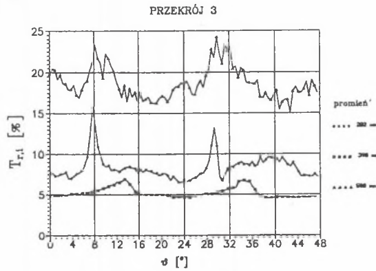
Rys. 8.4. Rozkład stopnia burzliwości
