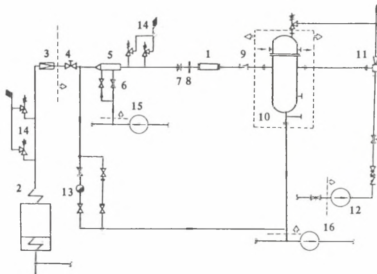
Rys. 9. Schemat instalacji tunelu parowego: 1) tunel parowy do badań palisadowych, 2) kocioł VELOX, 3) stacja redukcyjna na kotle, 4) zawór zaporowy, 5) stacja redukcyjno-schładzająca, 6) zawór regulujący dopływ skroplin do schładzacza, 7) zwężka pomiarowa, 8) kompensator soczewkowy, 9) przepustnica regulacyjna, 10) skraplacz, 11) strumienica wodna, 12) pompa wody roboczej dla strumienicy, 13) odwadniacz pływakowy, 14) zawory bezpieczeństwa, 15) pompa zasilająca, 16) pompa kondensatu
