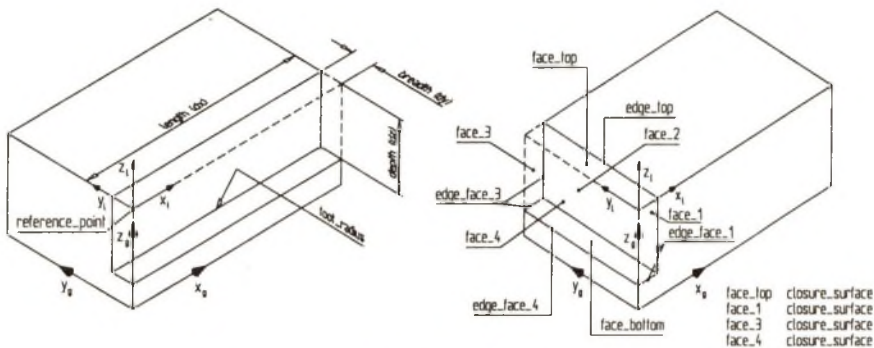
Bild 4: Stufe mit geometrischer Parameter- und Flächenbeschreibung
