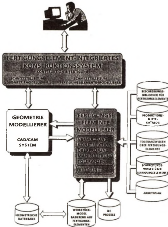
Bild 2. Architektur-Überblick von FINDES
