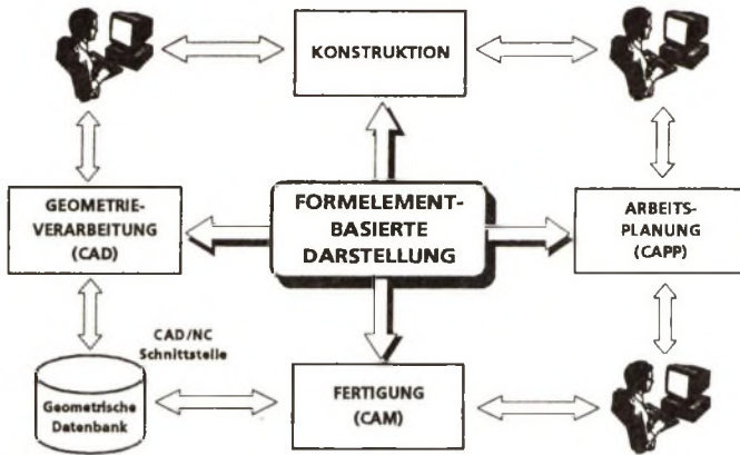
Bild 1. Übertragung der Informationen in CAD/CAPP/CAM-Systemen
