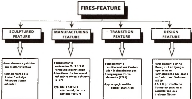
Bild 3. FIRES-feature Klassifizierung
